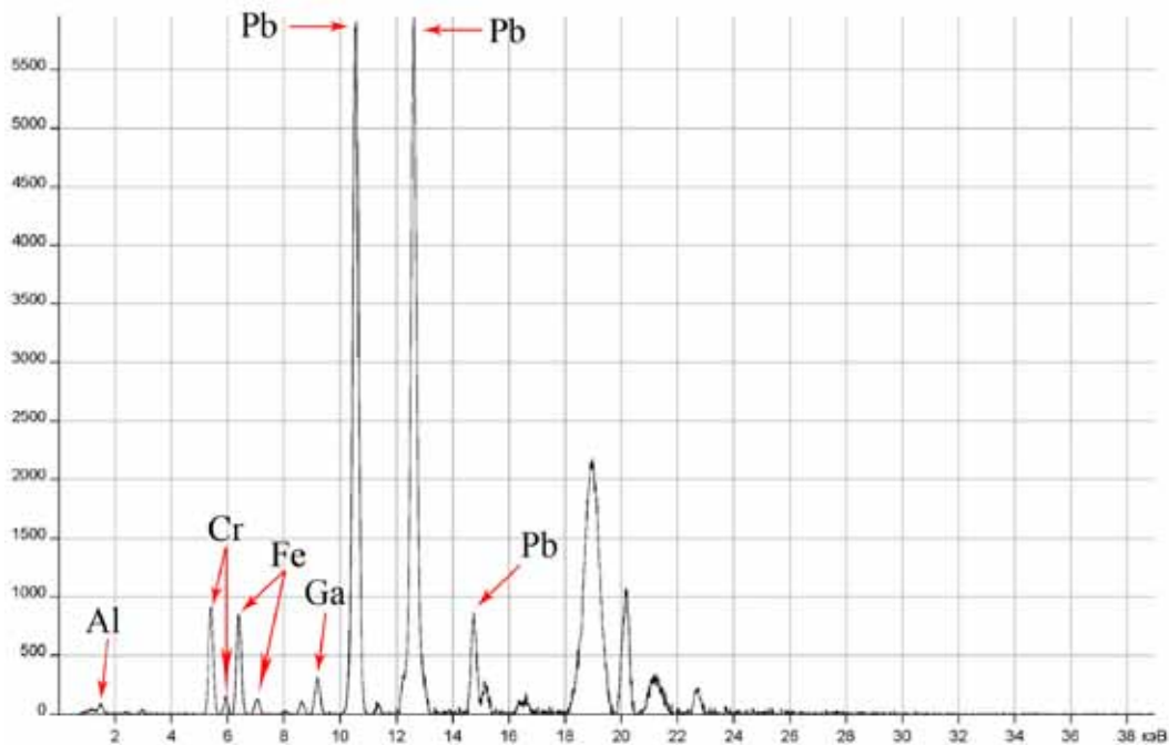
Рисунок 5. Рентгенівський спектр облагодженого рубіну
