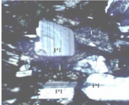
Рисунок 9. Фрагмент шліфа з кристалами плагіоклазу та ліпоїдними уламками вулканічного туфу. 1 – літоїдний уламок. Шліф Ол-27. Зображення під поляризаційним мікроскопом з введеним аналізатором. Розмір зображення 2x1,5 мм
